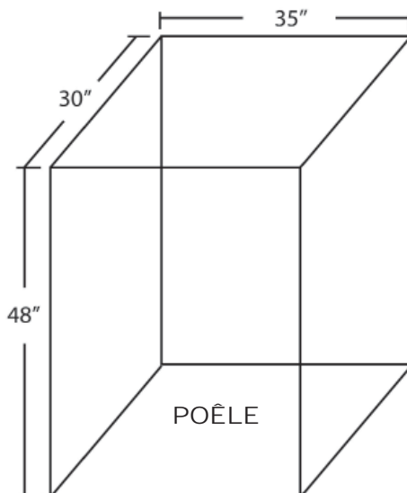
Dimensions minimales de l'alcôve
